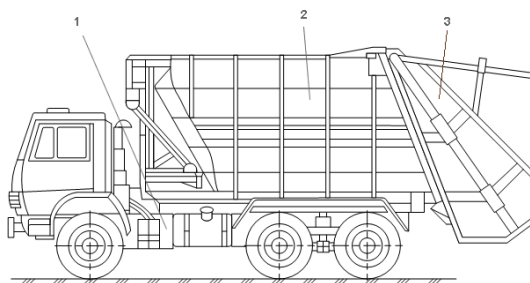
Рис. 4.28. Мусоровоз кузовной с задней загрузкой
