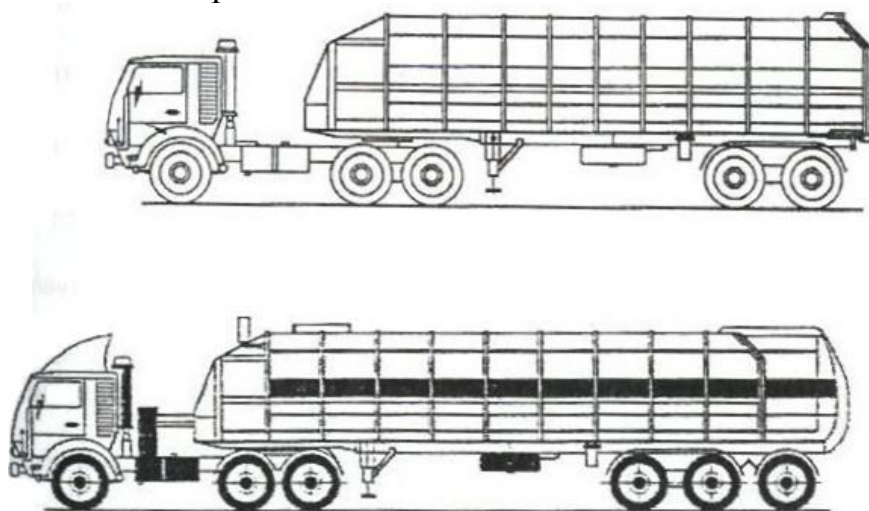
Рис. 4.23. Большегрузные транспортные мусоровозы МКТ-110, МКТ-150
