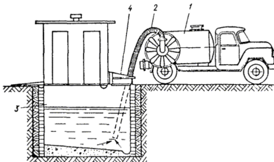
Рис. 5.6. Схема устройства выгреба для совместного сбора жидких и твердых бытовых отходов
