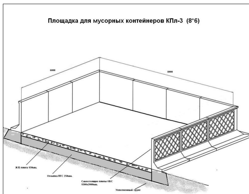
Рис. 4.17. Схема контейнерной площадки КПл-3 фирм ООО «Кавалер»
