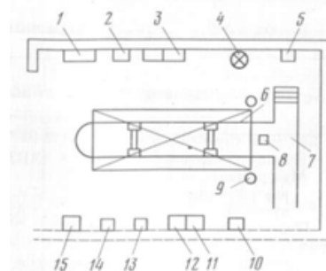
Рис. 7.2 Схема универсального поста ТО-2:
