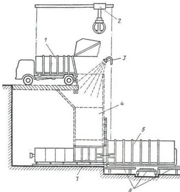
Рис. 4.25. Схема мусороперегрузочной станции с прессованием ТБО стационарным уплотнителем.
