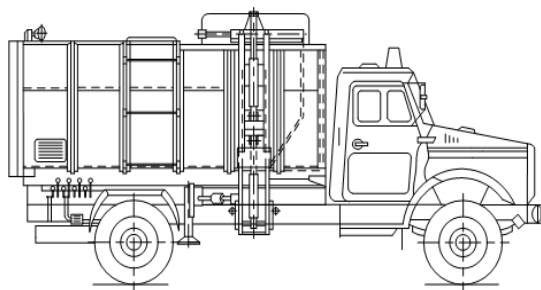
Рис. 4.29. Кузовной мусоровоз с боковой загрузкой кузова манипулятором
