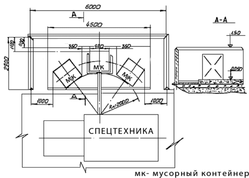
Рис. 4.14. Устройство контейнерной площадки
