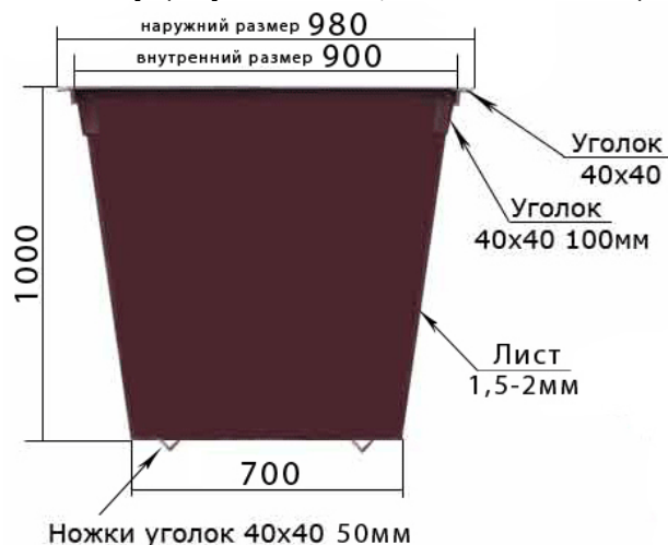
Рис. 4.10. Стандартные металлические контейнеры емкостью 0,75 м³
